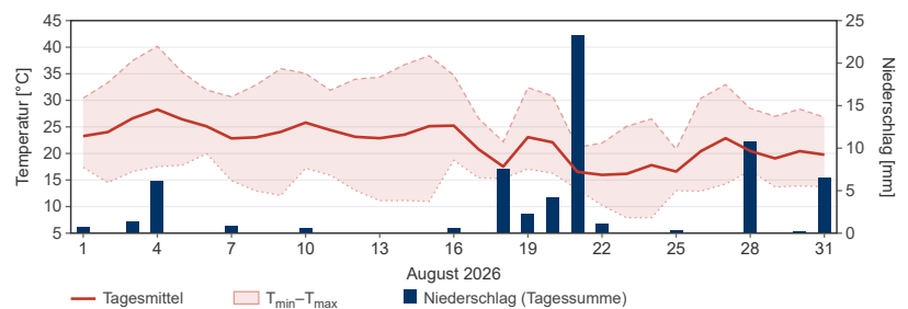
Lufttemperatur und Niederschlag, August 2026 (KU-Wetterstation Eichstätt).
