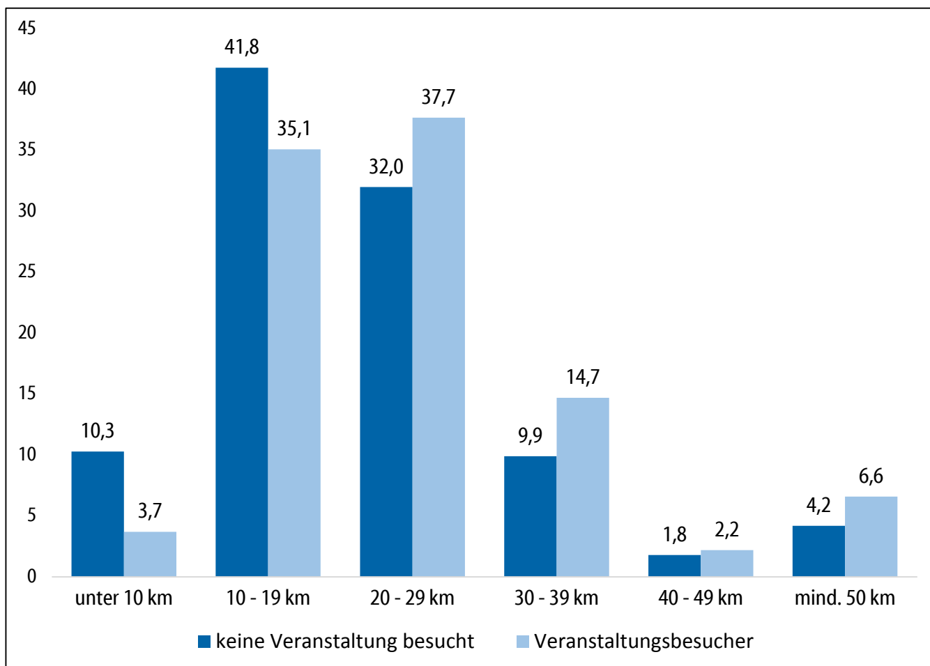
Abbildung 4: mögliche Fahrstrecke (N: Veranstaltungsbesucher=1976, keine Veranstaltung besucht=881)
